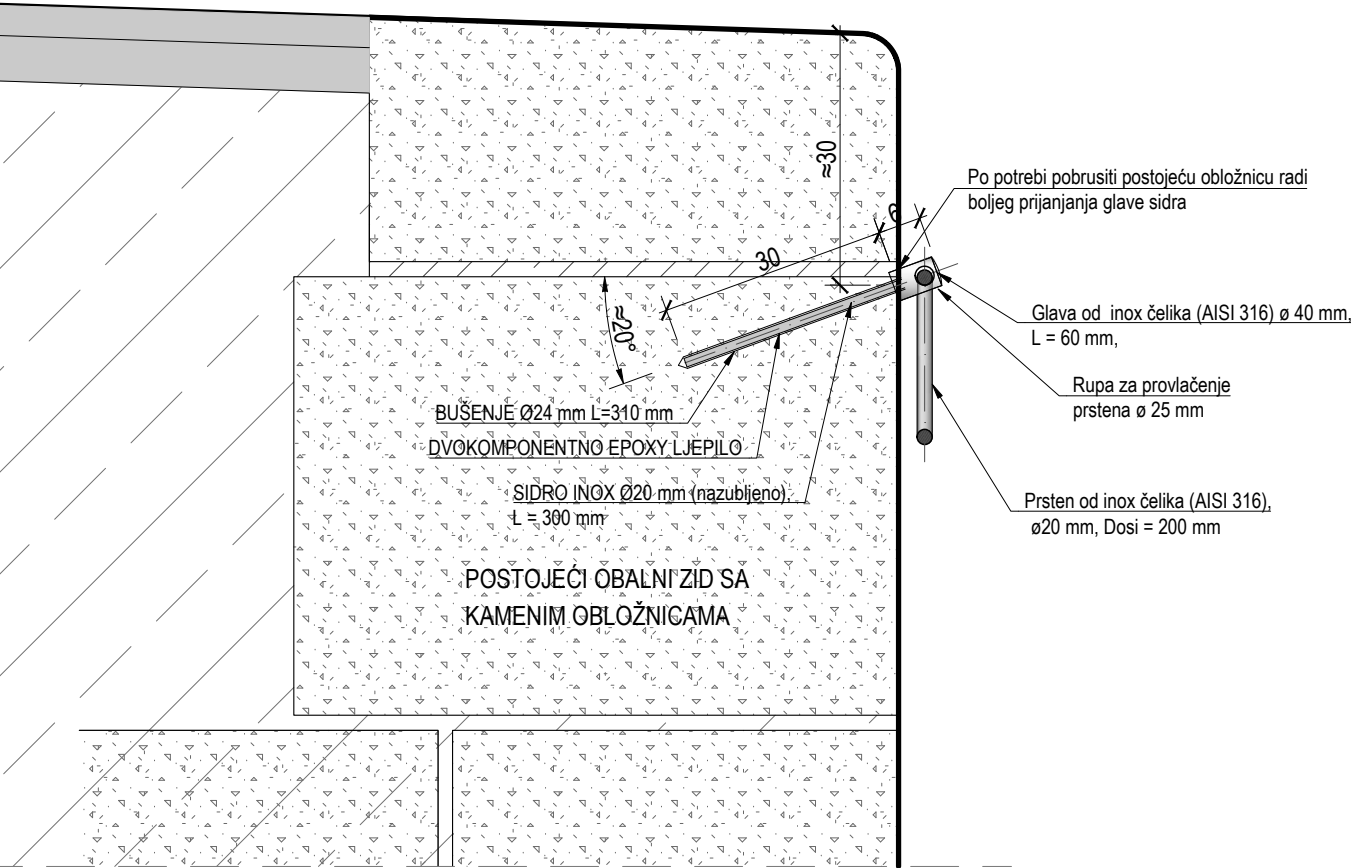
PRESJEK mj 1:10
