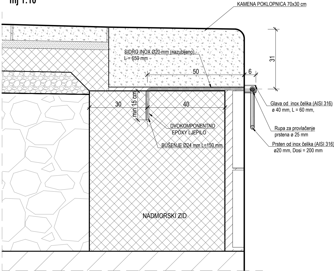
PRESJEK mj 1:10
